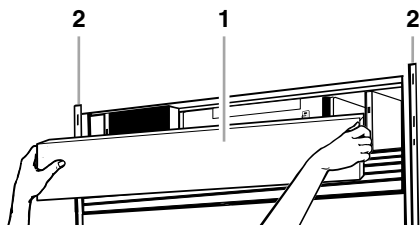
1. Rejilla superior 2. Adornos laterales del gabinete
